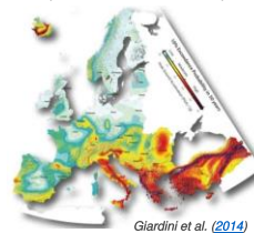
European Seismic Hazard Map
